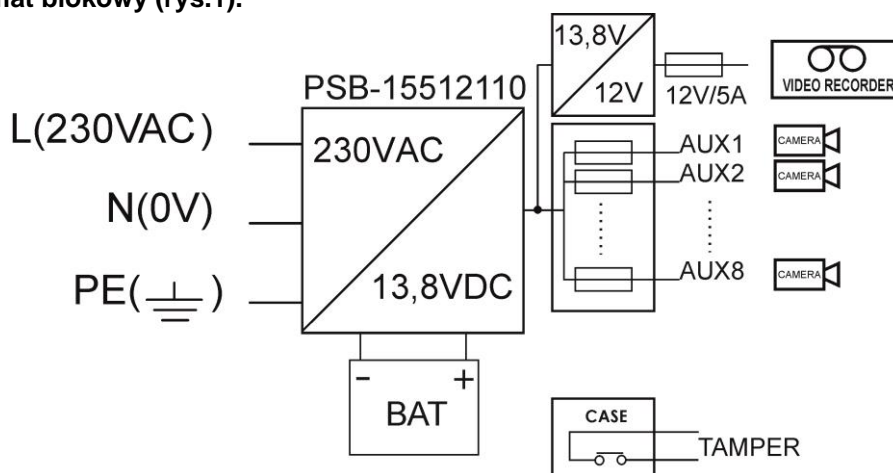
Rys.1. Schemat blokowy zasilacza.
